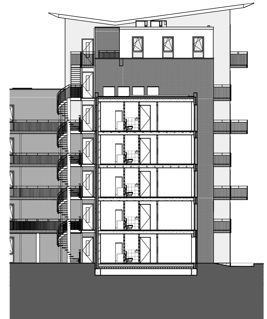
Doorsnede D-D
