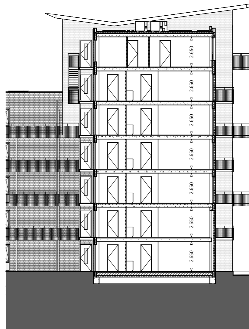
Doorsnede C-C
