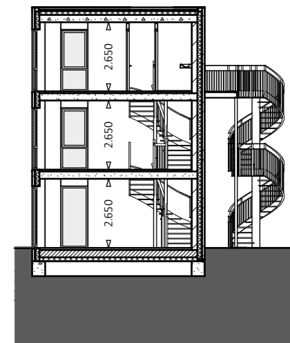
Doorsnede FF
