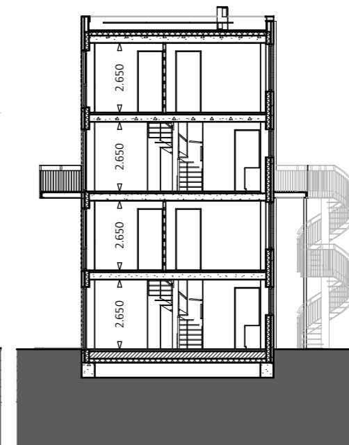
Doorsnede GG
