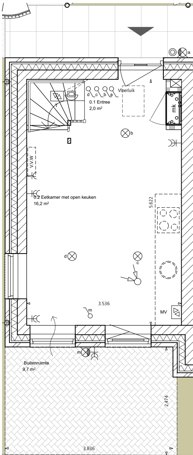
Begane grond
